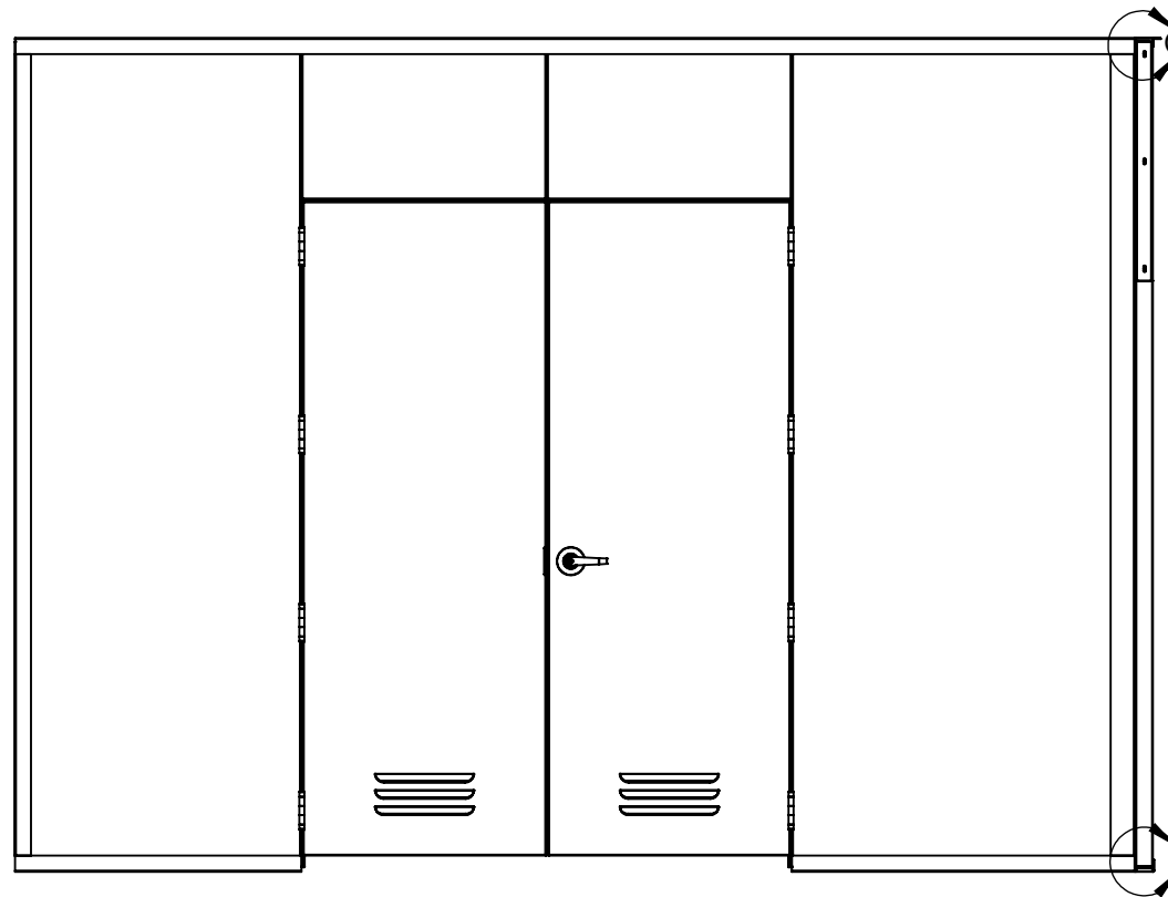
SECTION A-A SCALE 1 : 26
